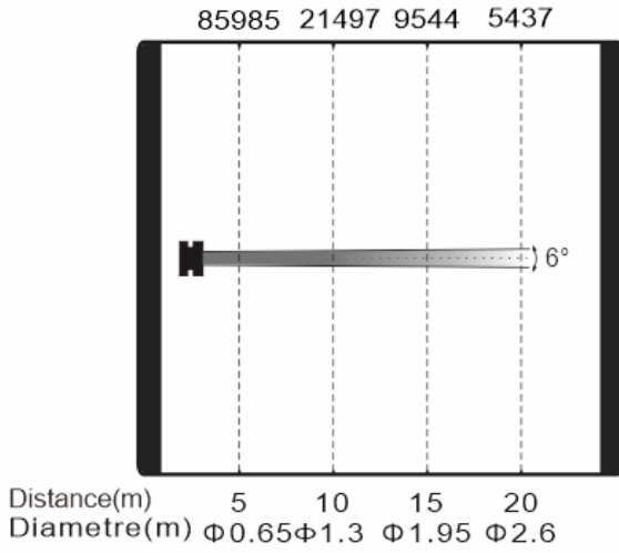
Min. Beam Mode Intensity LUX (6°)
